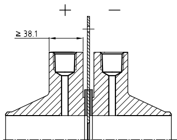
Flange tap
