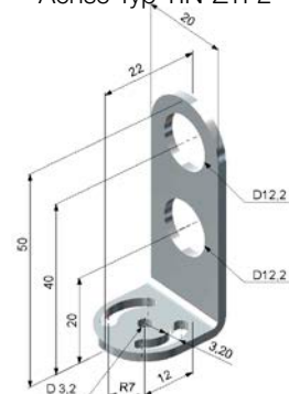
Montagewinkel, justierbar in einer Achse Typ TIN-ZTF2
