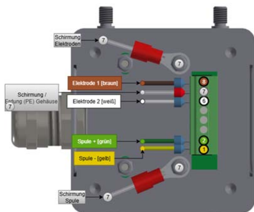
Anschlussbild Transmitter
