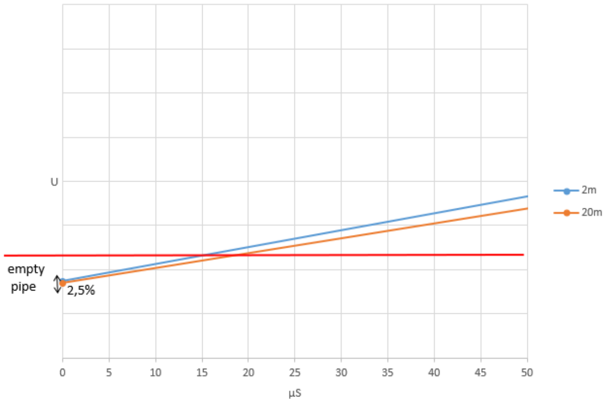
Einfluss Kabellänge und Leitfähigkeit auf verwertbare Messspannung
